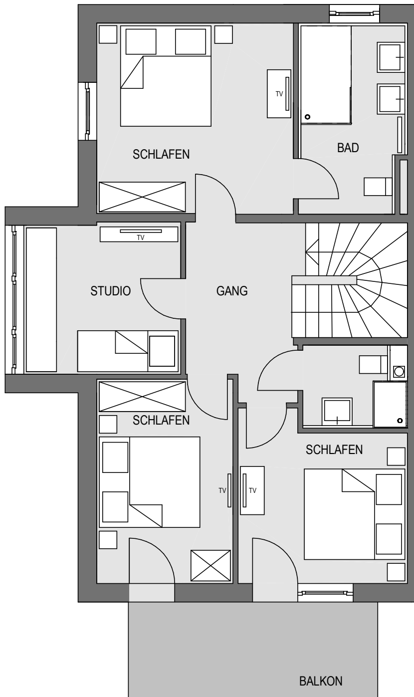
OBERGESCHOSS
